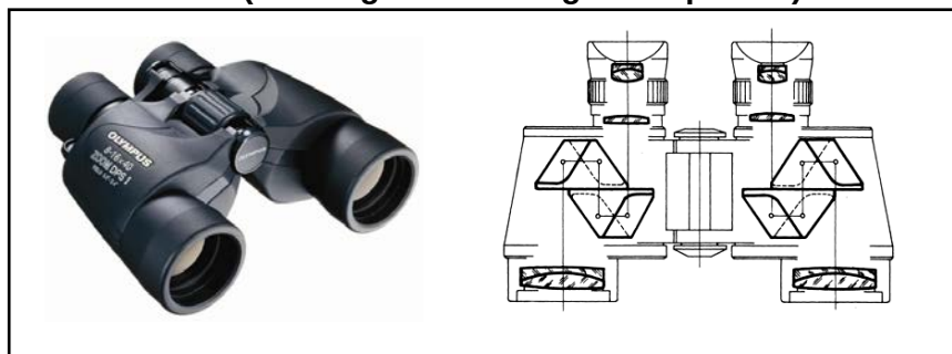
Binocolo (convergente + divergente + prisma)
